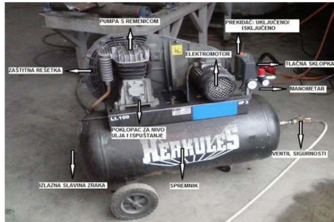
Gambar 2 : Kompresor
